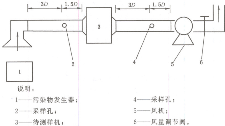
图 A.1 餐饮油烟净化设备示意图
